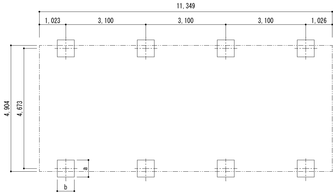
■基礎配置図
